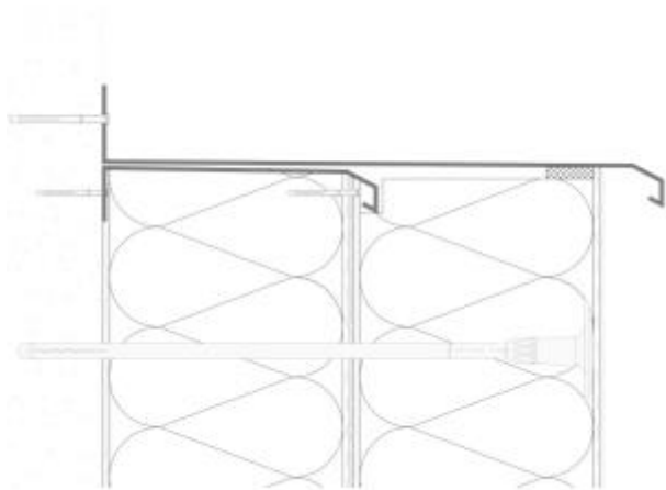
Figure 8a : nouvelle couverte inversée sans dépose de l'existant
