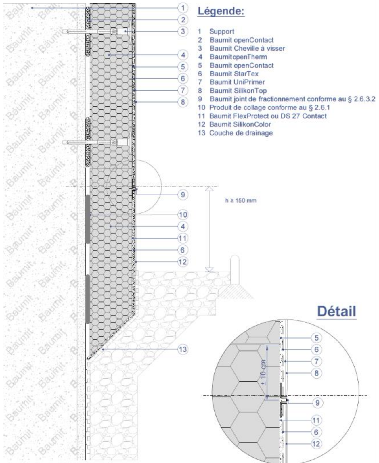
Figure 9c : départ en partie semi-enterrée coplanaire - partie semi-enterrée et partie courante au même nu Figure 9 : Départ en partie semi-enterrée
