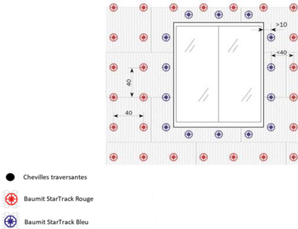
Figure 5a : Chevillage au niveau des baies sans augmentation du nombre de chevilles
