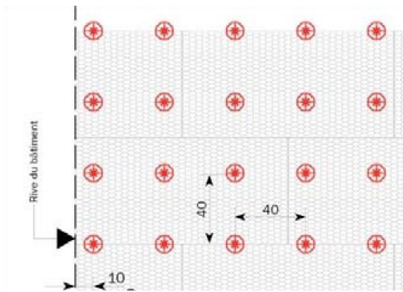
Figure 3a : Calepinage 40 cm x 40 cm
