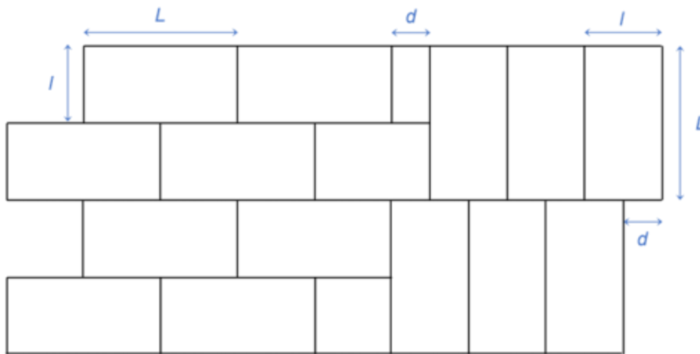
Figure 1 : Principe de juxtaposition des poses horizontale et verticale des panneaux isolants
