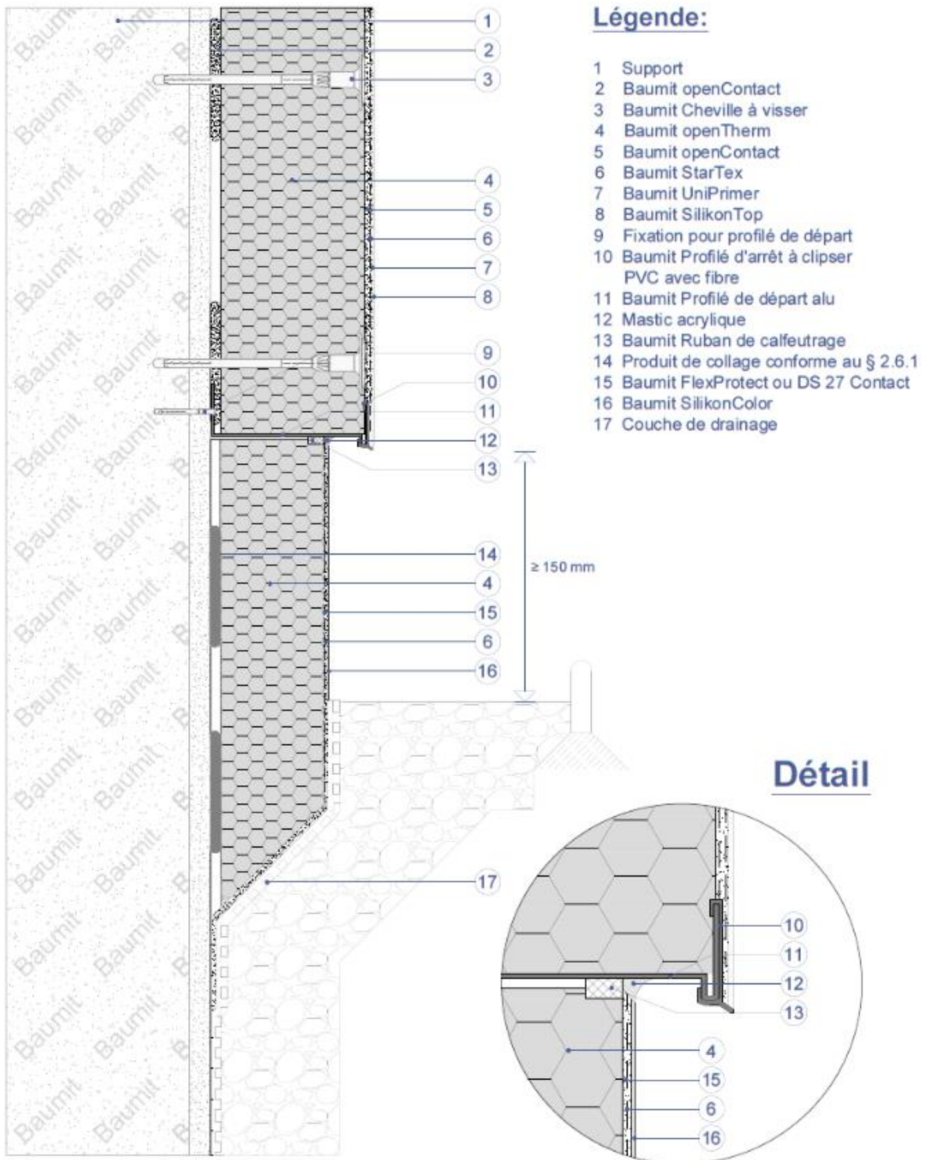
Figure 9a : Départ en parties semi-enterrées – décroché entre la partie enterrée et la partie courante
