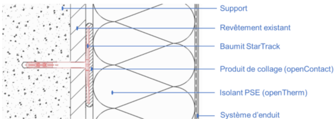
Figure 4 : Principe de fonctionnement du chevillage avec Baunit StarTrack
