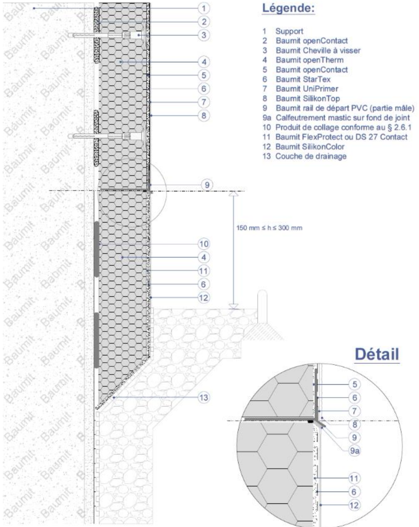
Figure 9b : départ en partie semi-enterrée coplanaire avec rail PVC - partie semi-enterrée et partie courante au même nu
